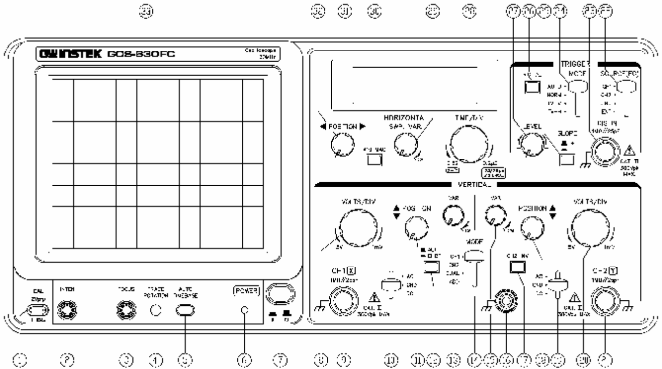
图 4-1 GOS-630FC 前面板
